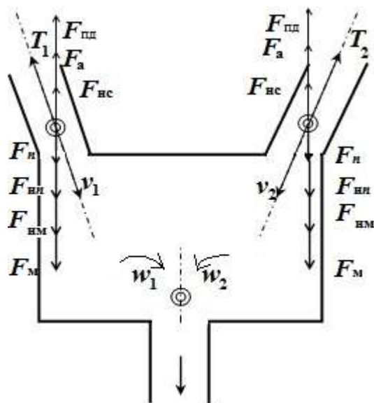
Рис. 1. Силы, действующие в газожидкостном потоке коллектора доильного аппарата
