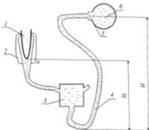
Рис. 2. Схема газожидкостного контура «молочная железа – доильный аппарат – молокопровод»: 1 – сосок вымени; 2 – доильный стакан; 3 – коллектор; 4 – молочный шланг; 5 – молочный кран; 6 – молокопровод
