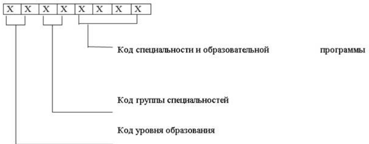
Рисунок 1 - Структура кодирования
